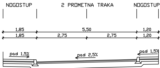
PRESJEK 1-1, MJ 1:100
