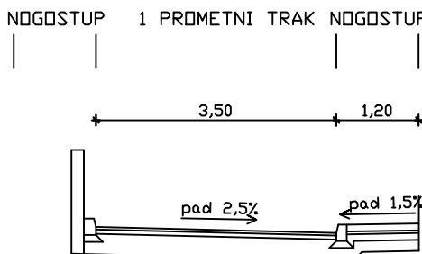
PRESJEK 2-2, MJ 1:100
